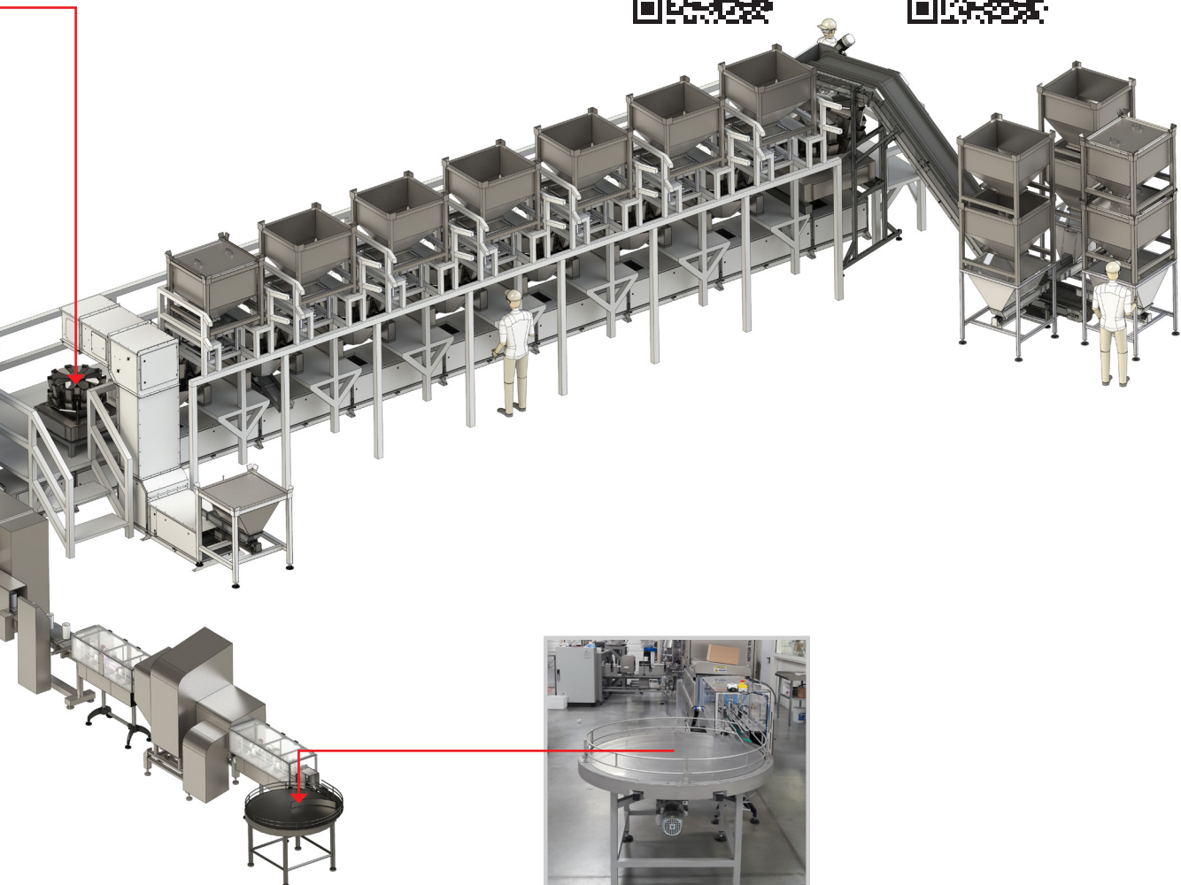
Otočný stůl OS
