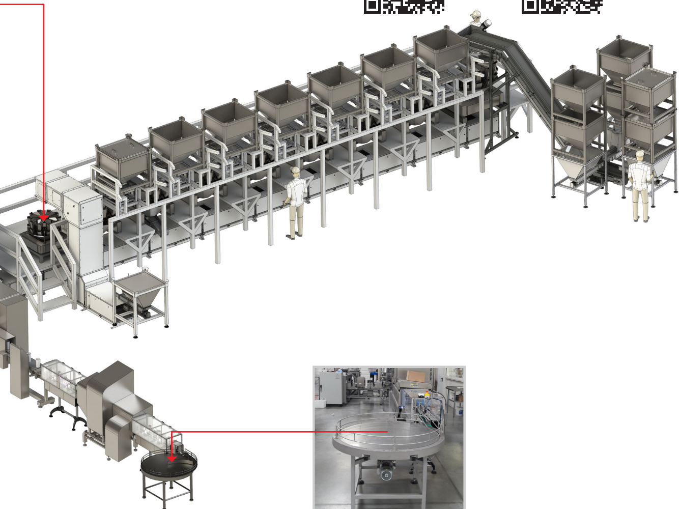
Rotating table OS
